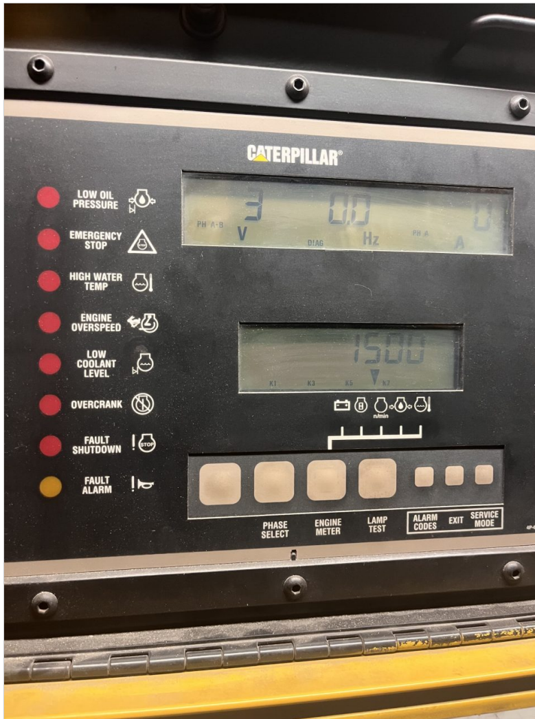
Verificación del equipo entregando 3 volts
