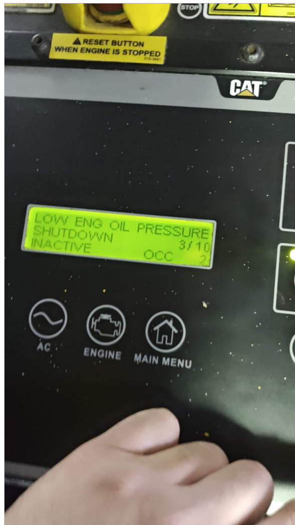
Proteccion por baja presion de aceite
